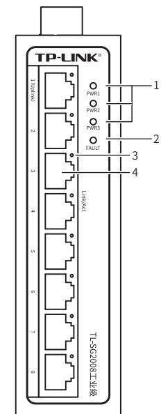
TL-SG2008工业级 前面板示意图
