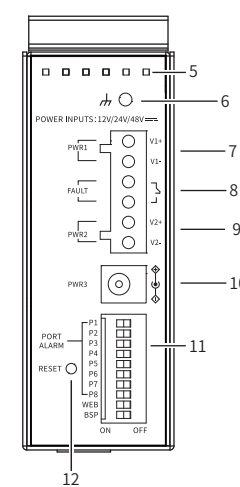
TL-SG2008工业级 上面板示意图
